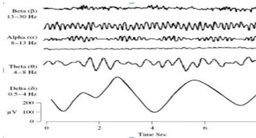
Grafik 1. Gelombang Otak Dari Delta Hingga Beta
